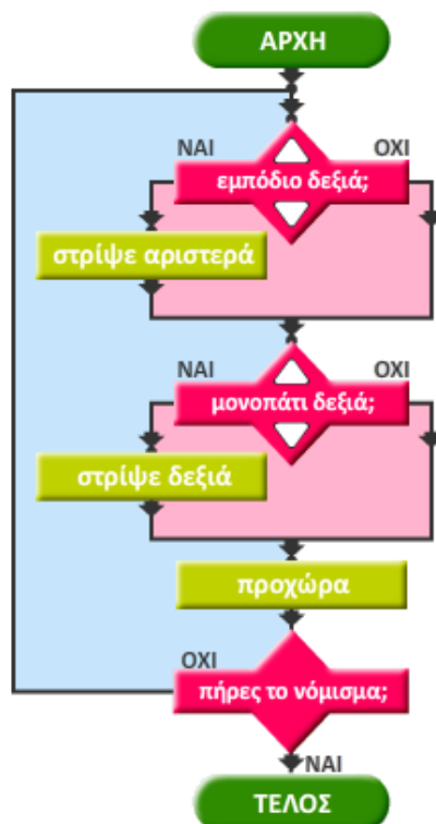
Σχήμα 3.29: Διάγραμμα ροής του κώδικα.
