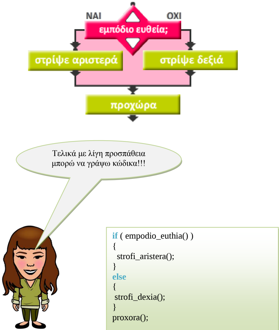
Σχήμα 3.38: Διάγραμμα ροής και κώδικας σε γλώσσα C.
