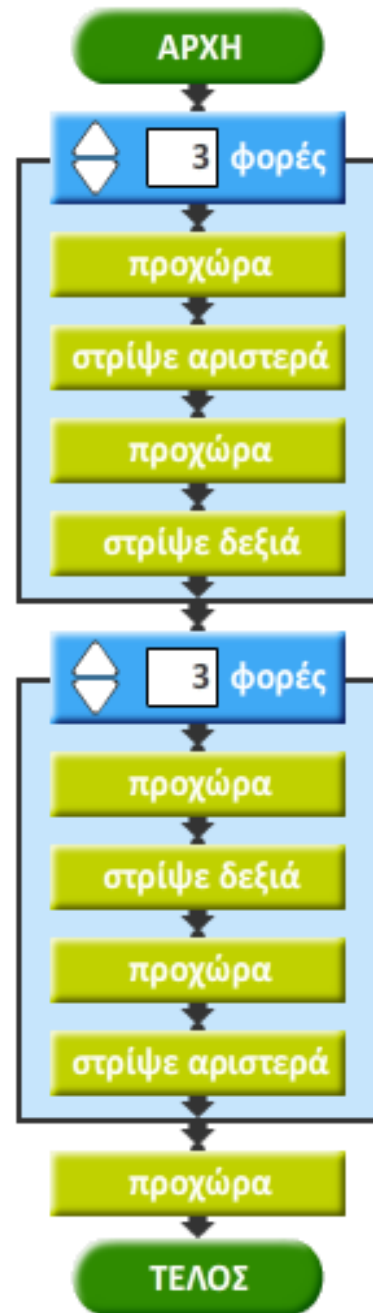
Σχήμα 3.35: Διάγραμμα ροής του κώδικα.
