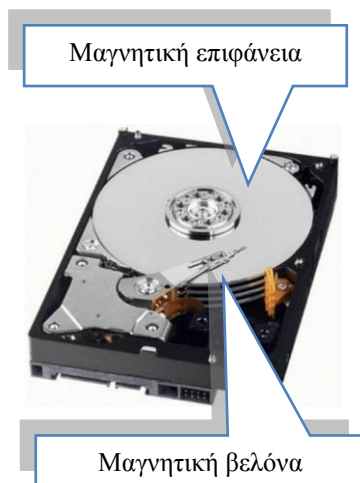
Σχήμα 2.2: Εσωτερικό σκληρού δίσκου.
